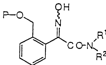
( II-1 )
