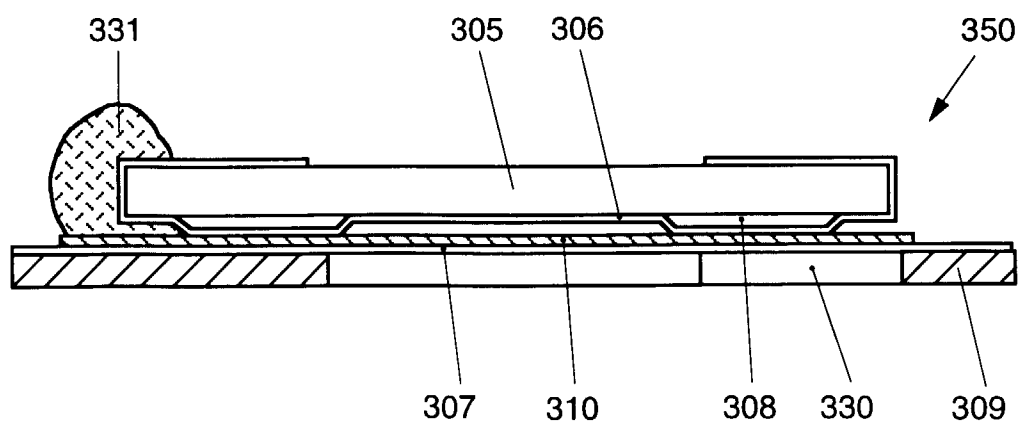
FIG. 3C
