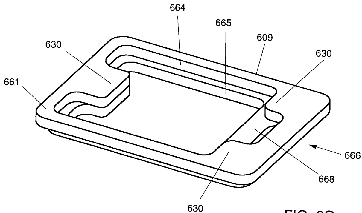
FIG. 6G
