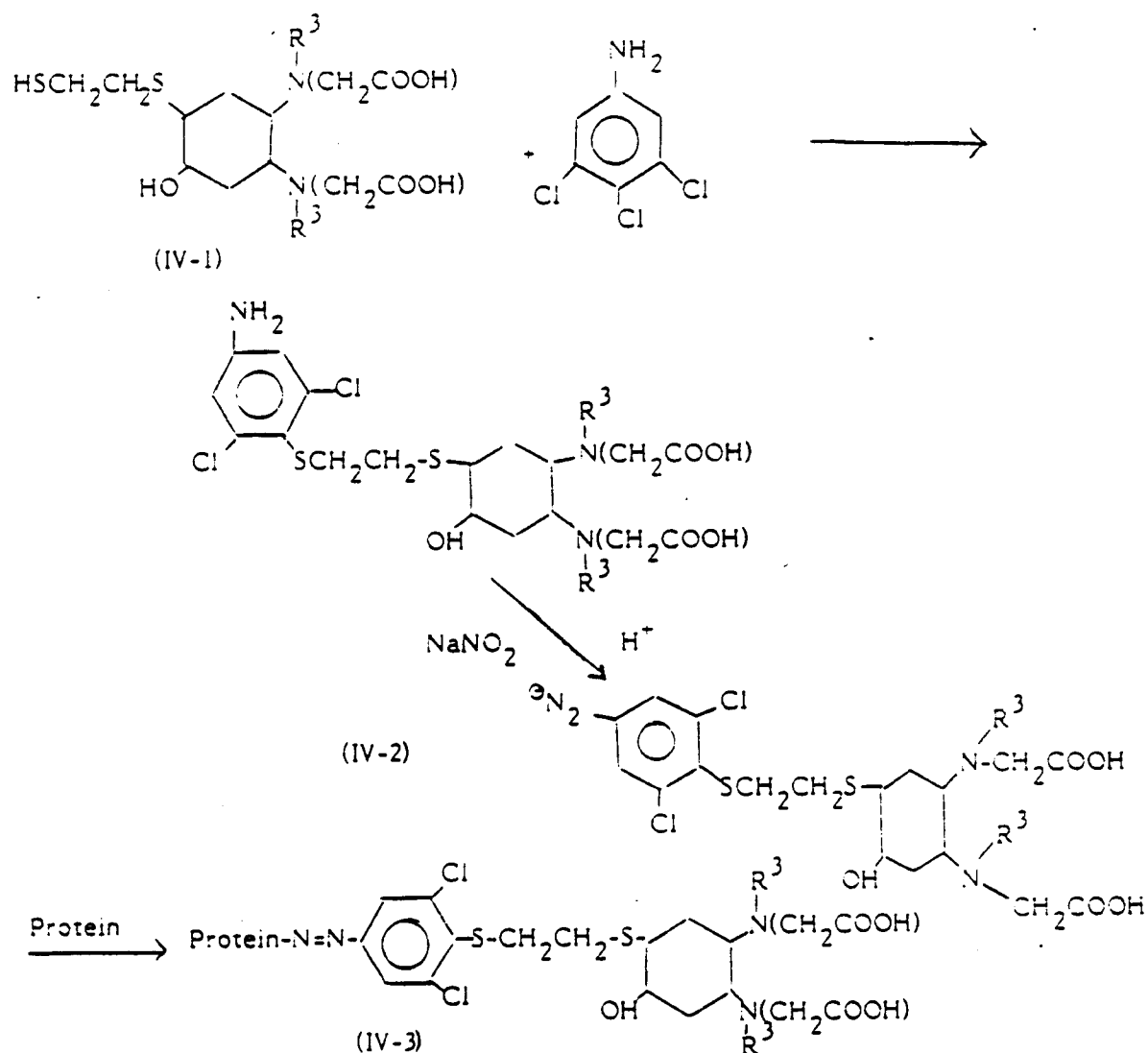
Scheme IV:
