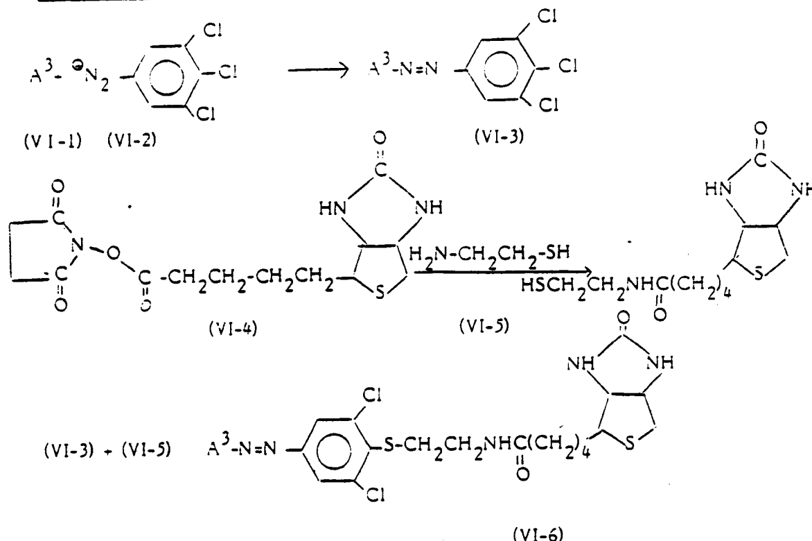
Scheme VI:
