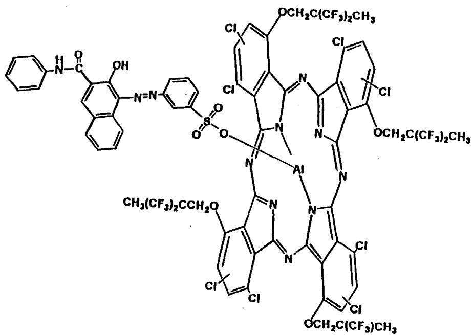
Phthalocyanine compound (d)
