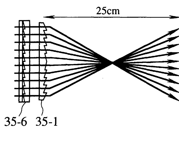
FIG.35B
