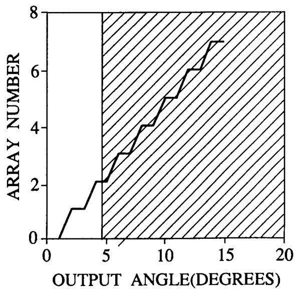
FIG.14C
