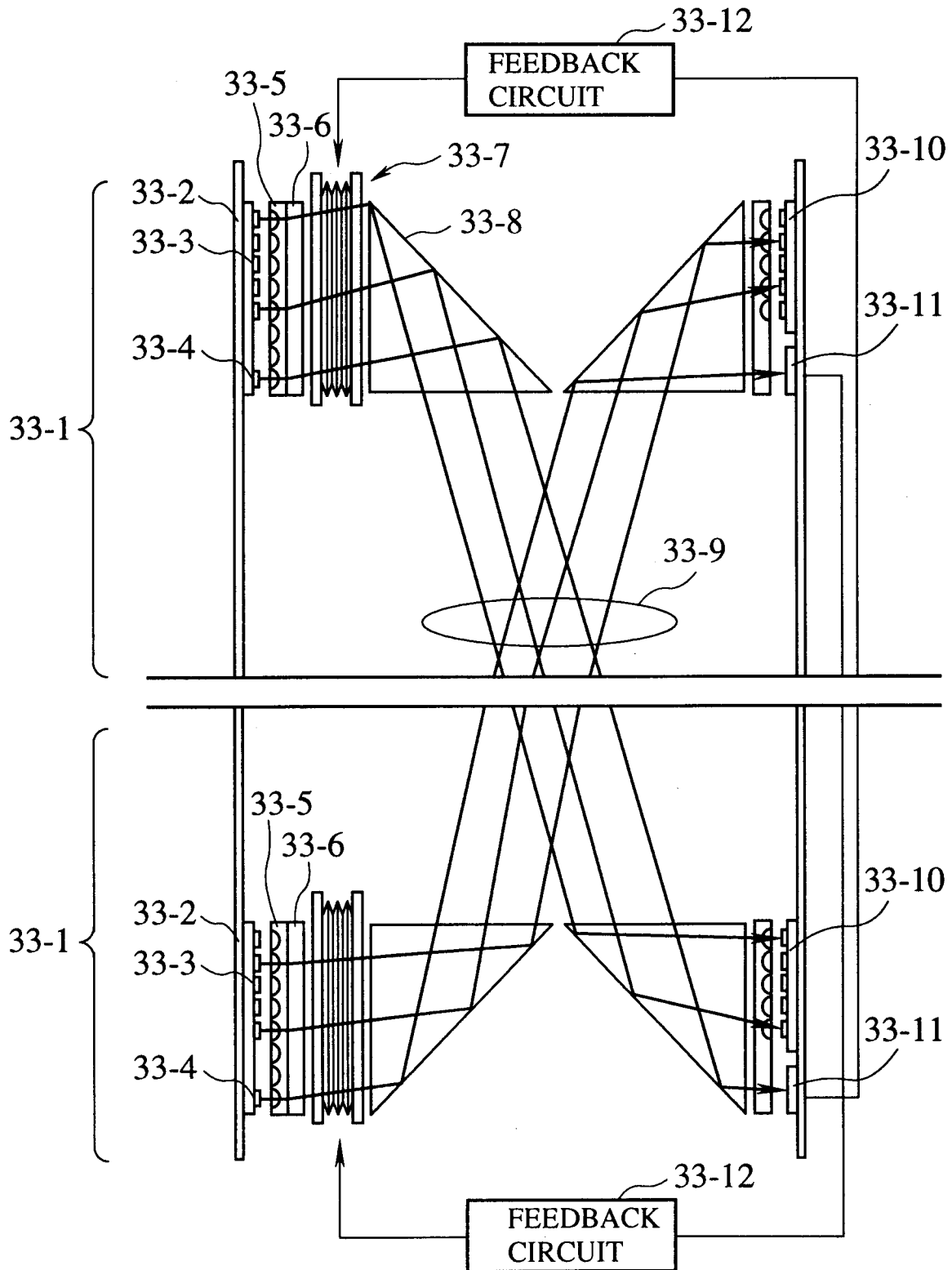
FIG.33
