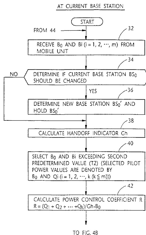
FIG. 4A
