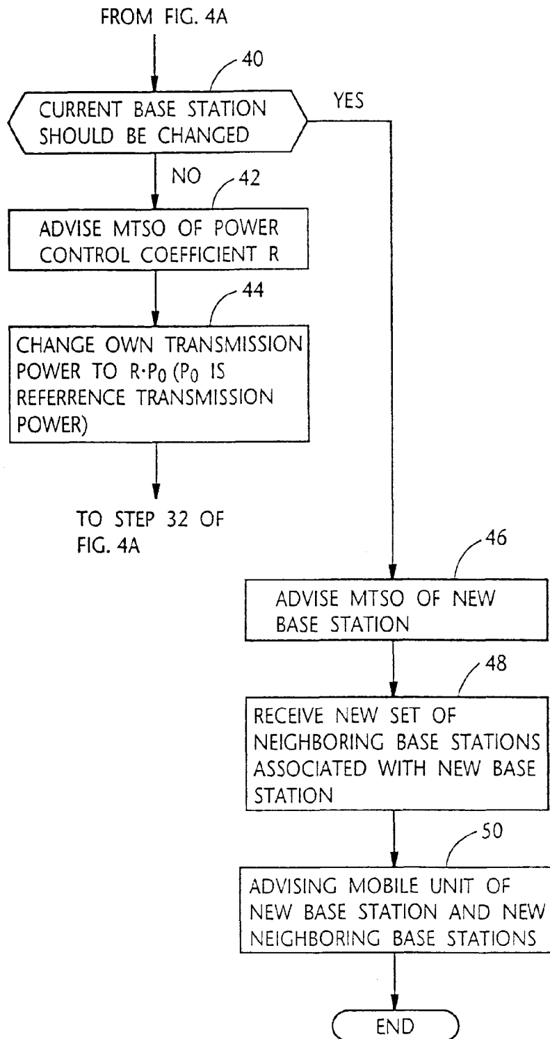
FIG. 4B
