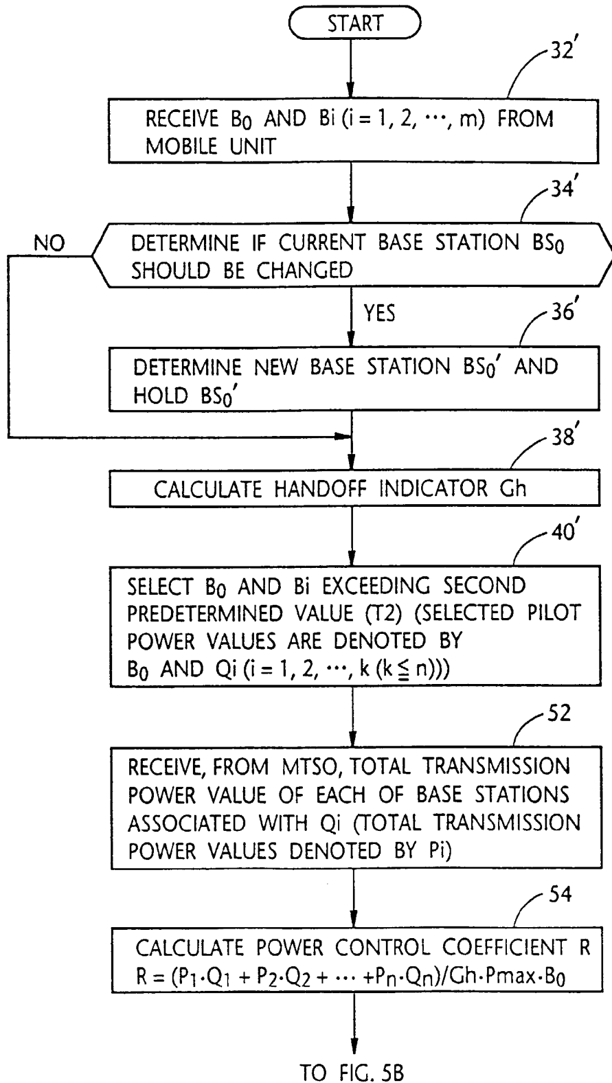
FIG. 5A
