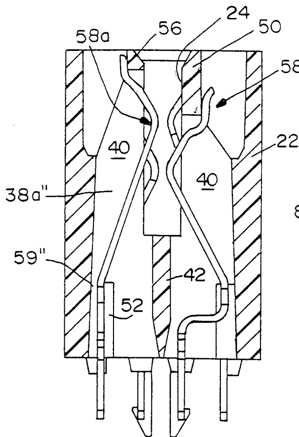
FIG. 19
