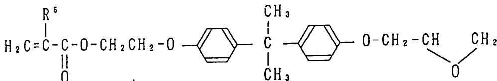
2-(4'-glycidyloxyphenyl)-2-[4'-(meth)acryloxyethoxyphenyl]propane
