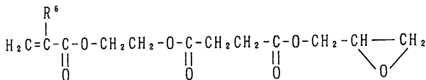
2-(4'-glycidyloxyphenyl)-2-[4'-(meth)acryloxyethoxyphenyl]propane
