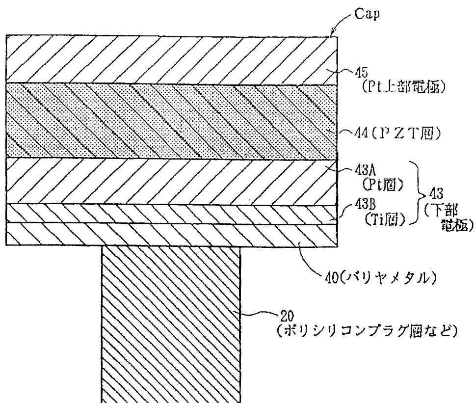
従来の P Z T キャパシタの構造
