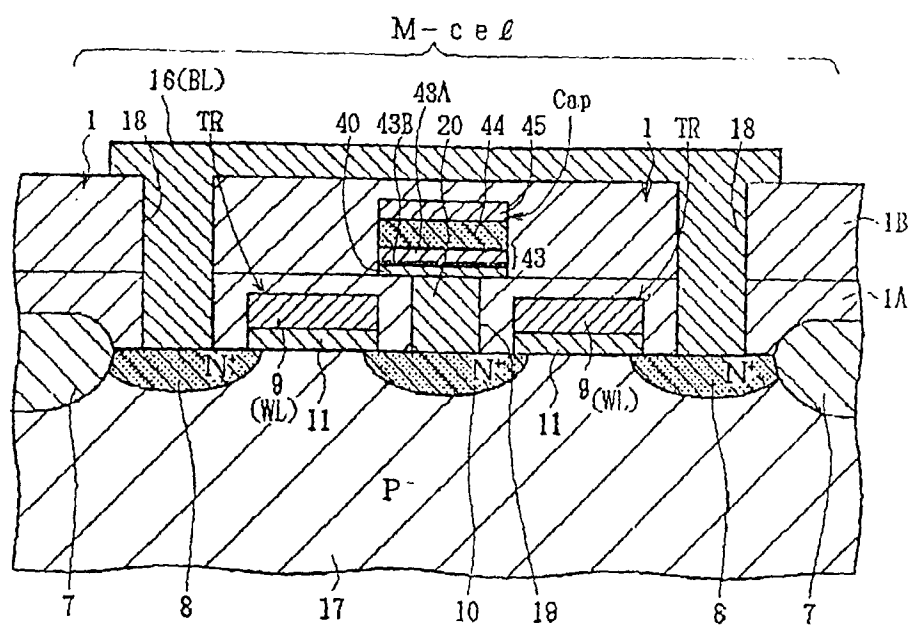
従来のデバイス断面構造
