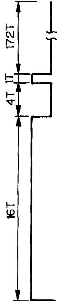
Fig. 2E REPETITION CODE RP
