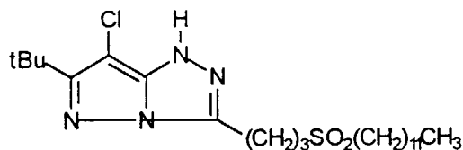
Cyan dye-forming coupler COUP-3
