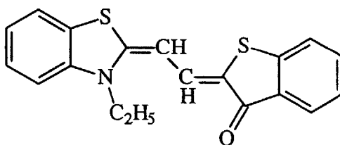
Magenta Dye M-2 "NK-1584"
