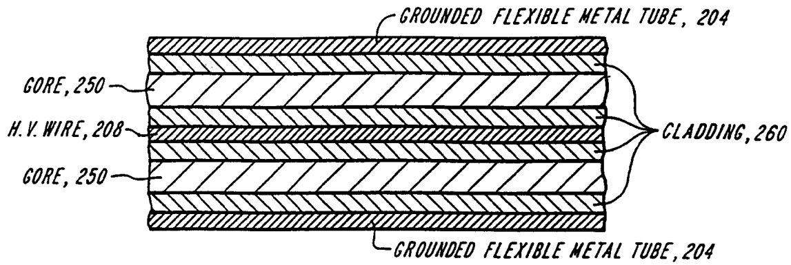
FIG. 20B
