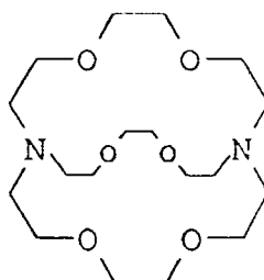
4,7,13,16,21,24-hexaoxa 1,10-diazabicyclo [8,8,8]- hexacosane of formula (D)
