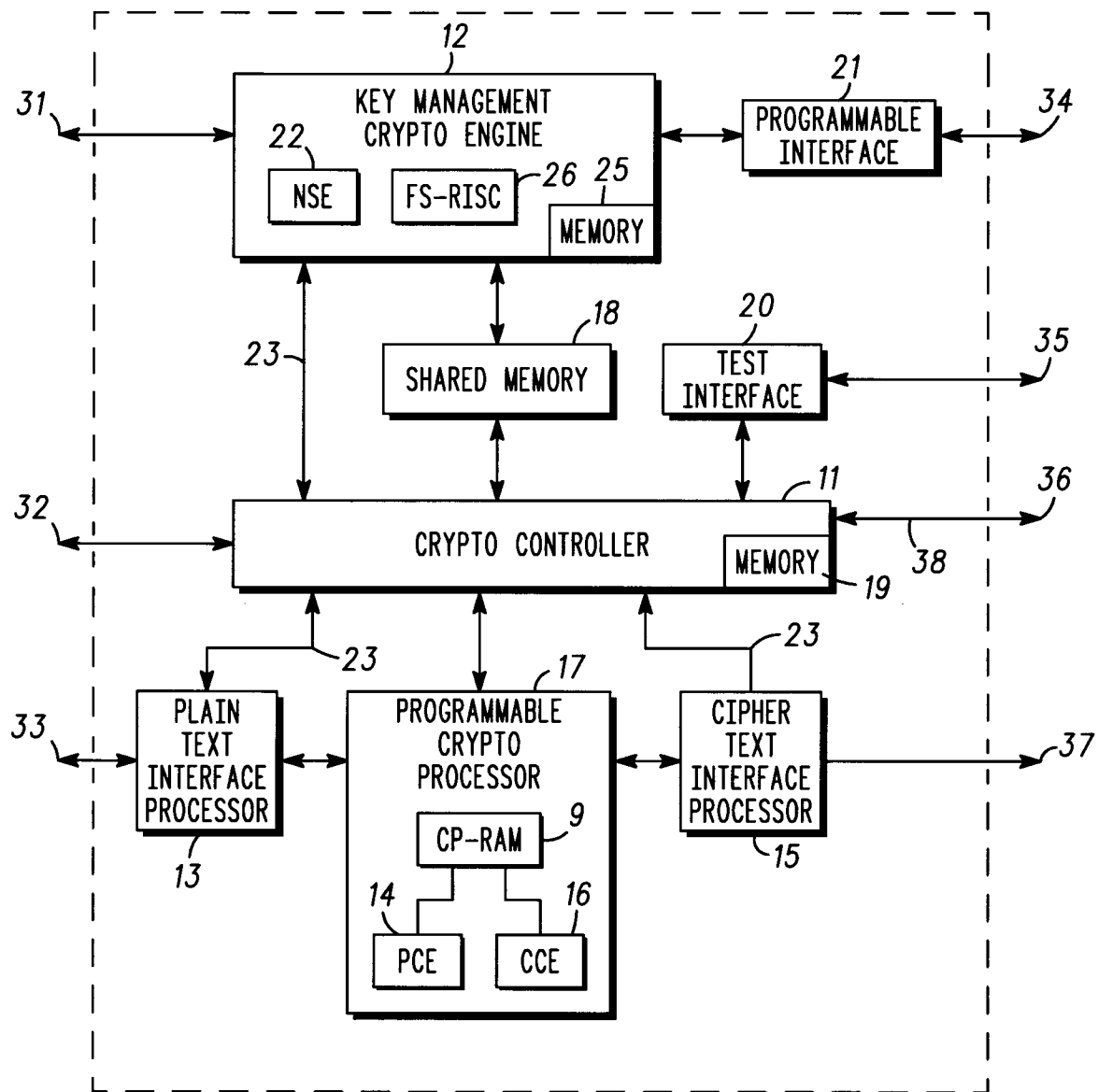
10 FIG. 1
