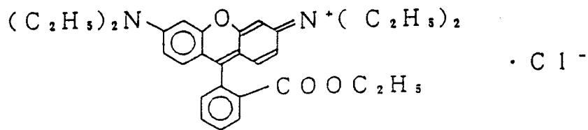
RHODAMINE 3 B
