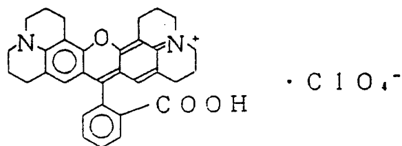
RHODAMINE 101
