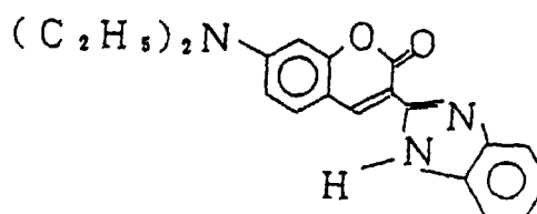
COUMARIN 7
