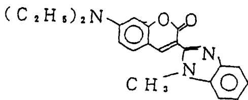
COUMARIN 30
