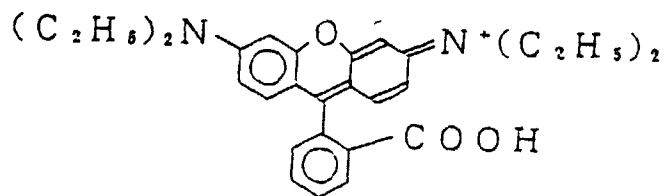
RHODAMINE B
