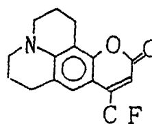
COUMARIN 153
