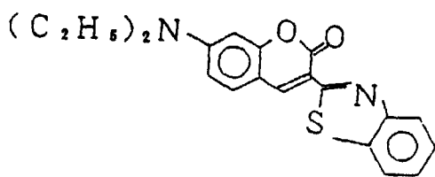
COUMARIN 6
