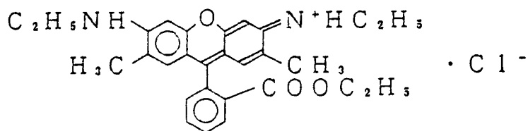
RHODAMINE 6 G
