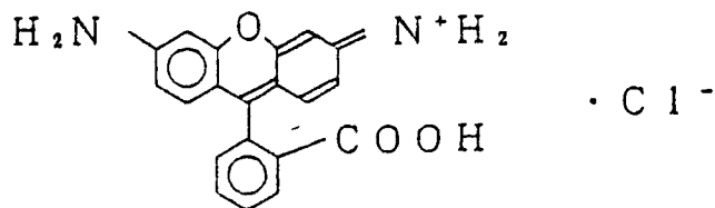
RHODAMINE 110
