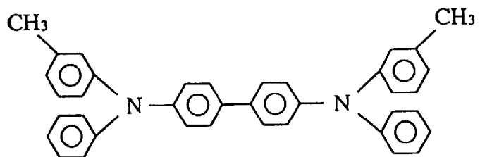
TPD
