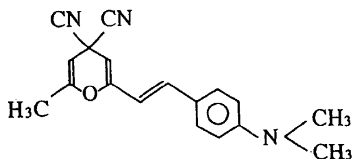
DCM
