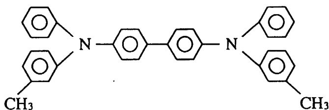
TPD
