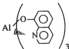
Alq 3
