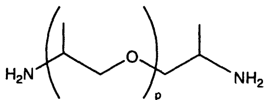
JEFFAMINE D230
