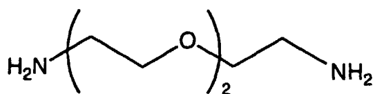
JEFFAMINE EDR148
