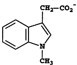
Cpd. 46
