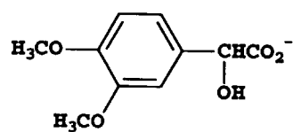
Cpd. 51
