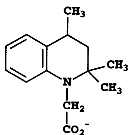
Cpd. 47
