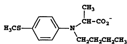
Cpd. 59
