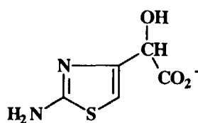
Cpd. 60
