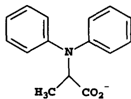
Cpd. 58
