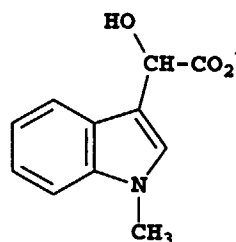
Cpd. 43
