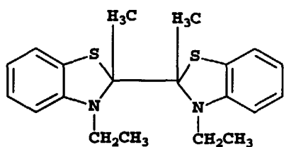
Cpd. 52
