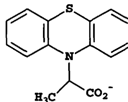
Cpd. 57
