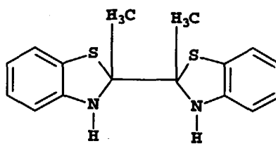
Cpd. 53
