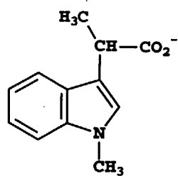
Cpd. 45
