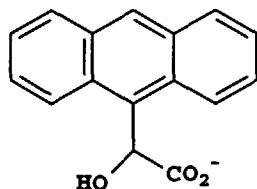
Cpd. 56
