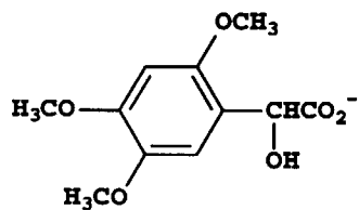
Cpd. 48
