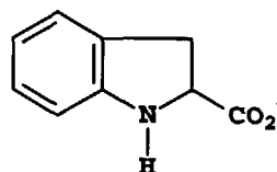
Cpd. 55
