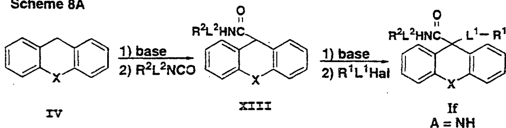
Scheme 8A
