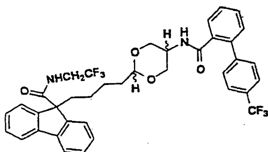
Isomère A
