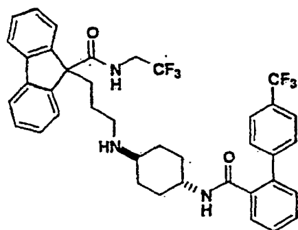
Isomère trans
