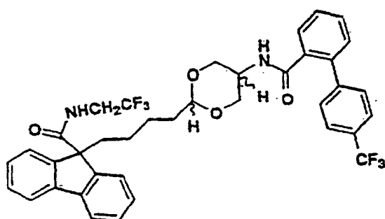
Isomère B
