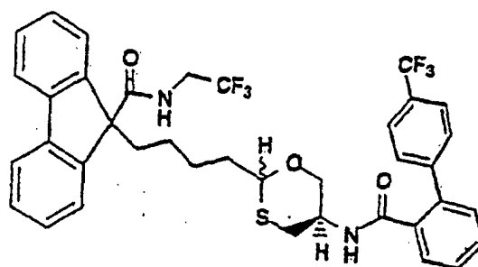
Isomère A
