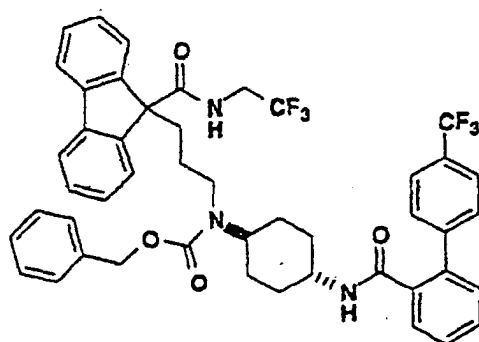
Isomère trans
