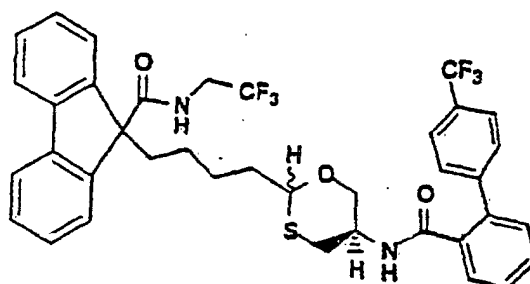
Isomère B
