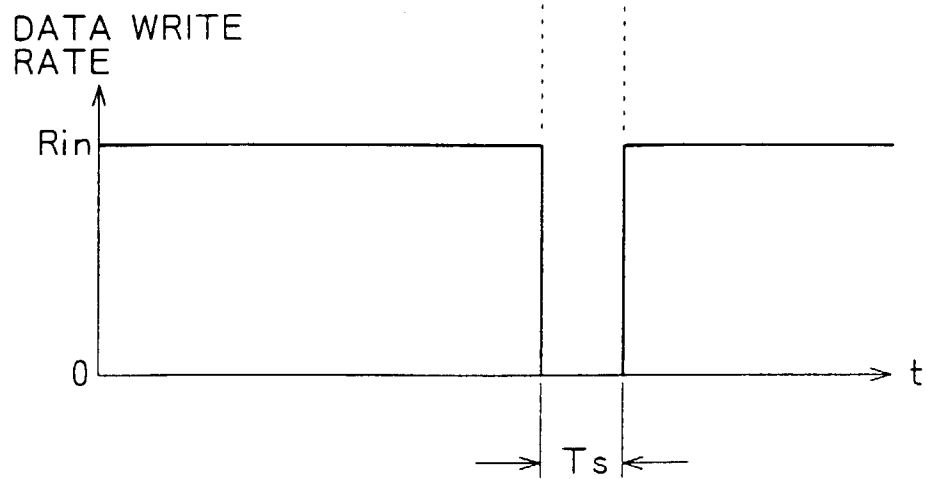
FIG. 20B
