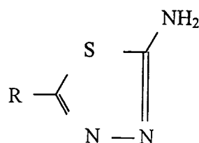
thiosemicarbazide
