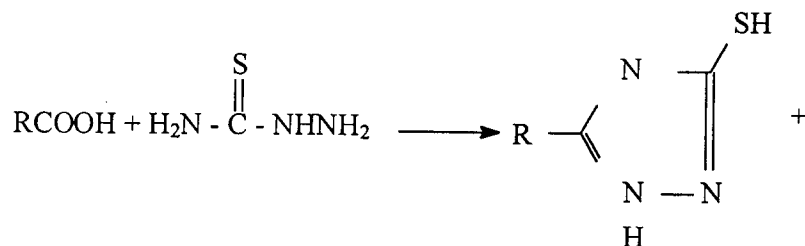
thiosemicarbazide
