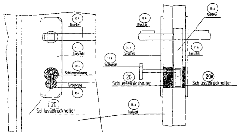
Fig. 1 Seitenansicht
