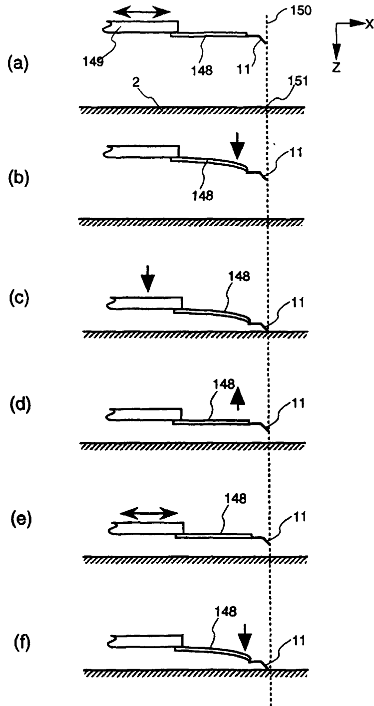
FIG.29
