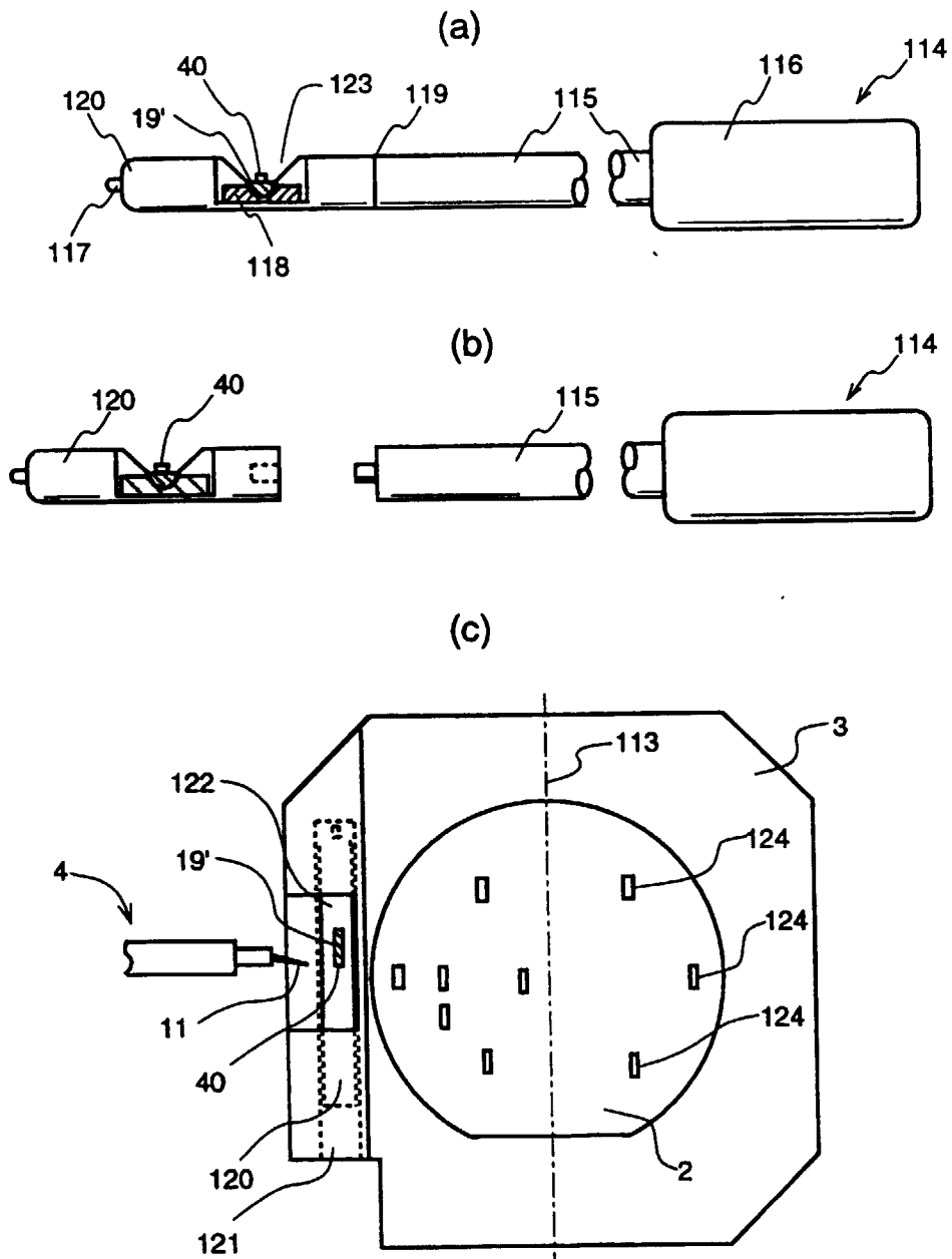
FIG.23
