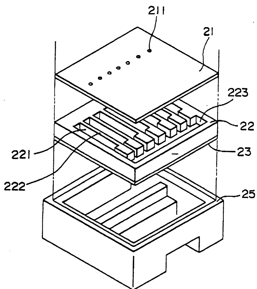
2: INK-JET PRINT HEAD
