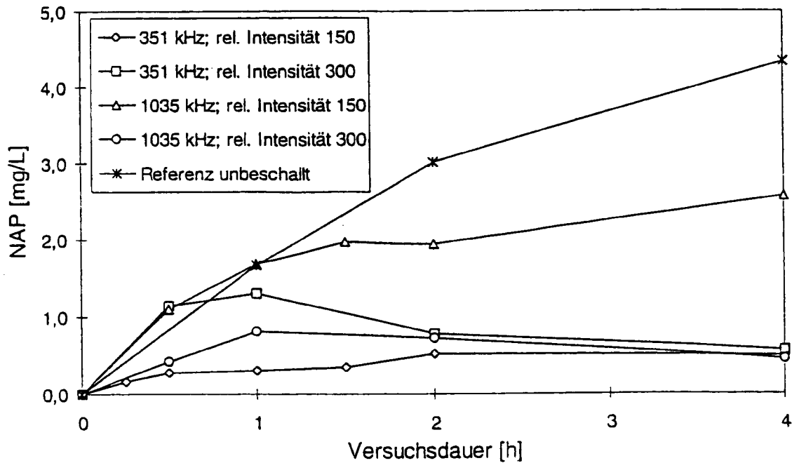
Fig. 3: Anstieg der UV-Absorption in der Wasserphase bei Beschallung von kristallinem Phenanthren (200 ppm) mit Ultraschall der Frequenzen 351 kHz und 1035 kHz bei unterschiedlichen Ultraschall-Intensitäten.
