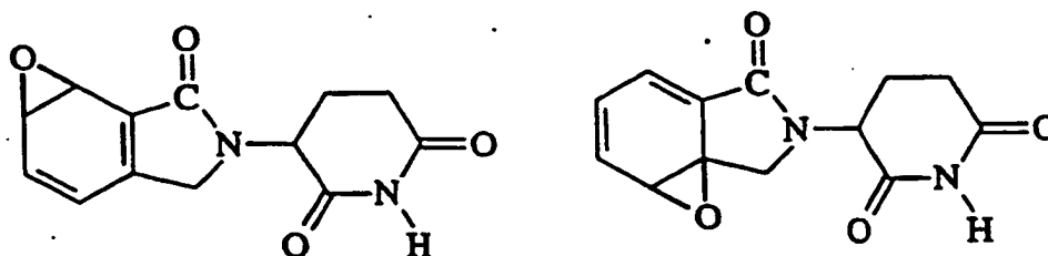
Epoxides of EM 12
