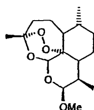
Artemether 3
