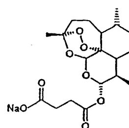
Sodium Artesunate 4
