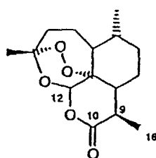
Artemisinin 1
