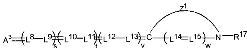
VI
