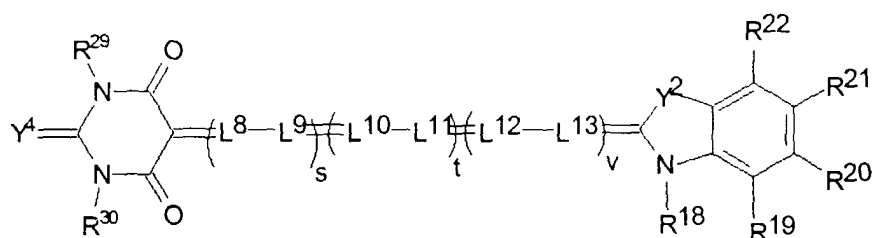
VIII-F
