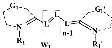
Ic
