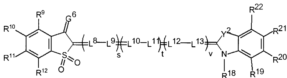
VIII-B
