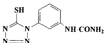
A-5
