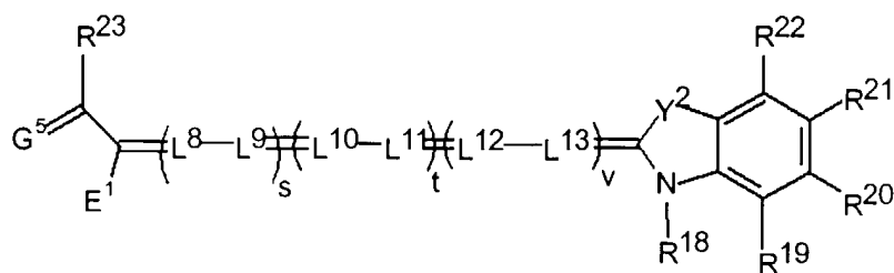
VIII-A
