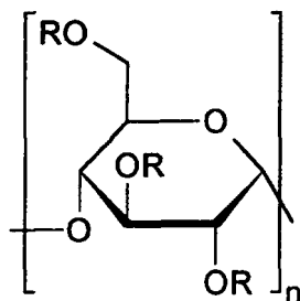
Strukturformel (I)
