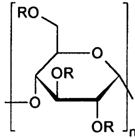
Strukturformel (I)
