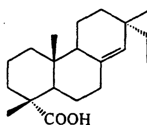
Sandaracopimaric 8
