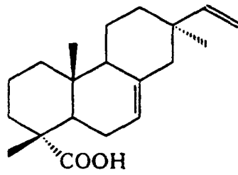
7,15-Pimaradienoic 10
