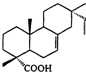
Isopimaric 7
