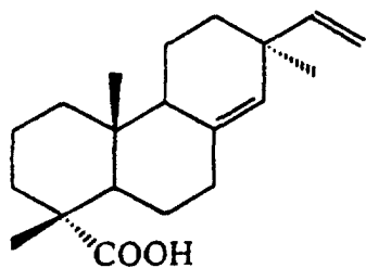
Pimaric 6
