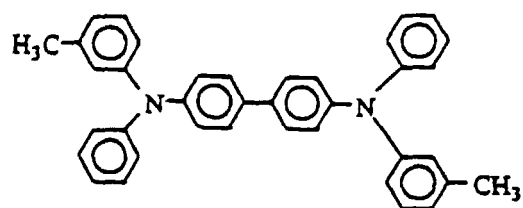
TPD
