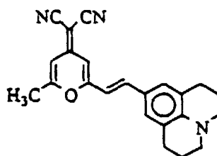
DCM2
