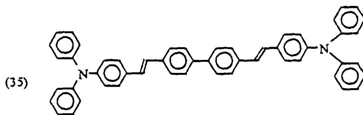
DSBi
