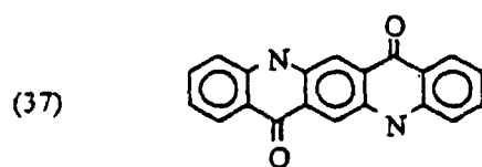
QNI
