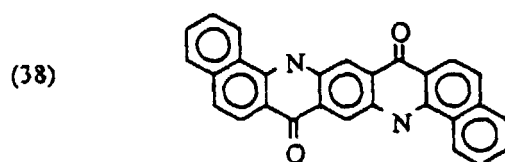
QN2
