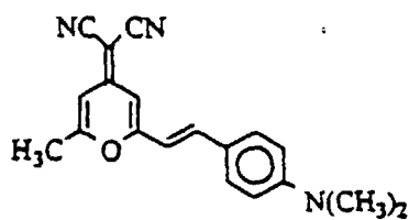
DCM1
