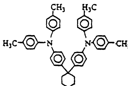
TPAC
