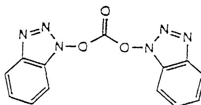
Di(1-benzotriazolyl) carbonate
