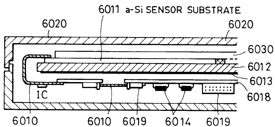
FIG. 18B
