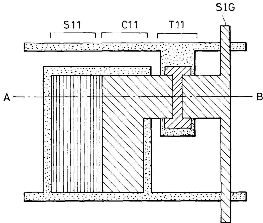
FIG. 17A
