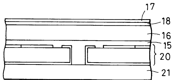
FIG. 16B
