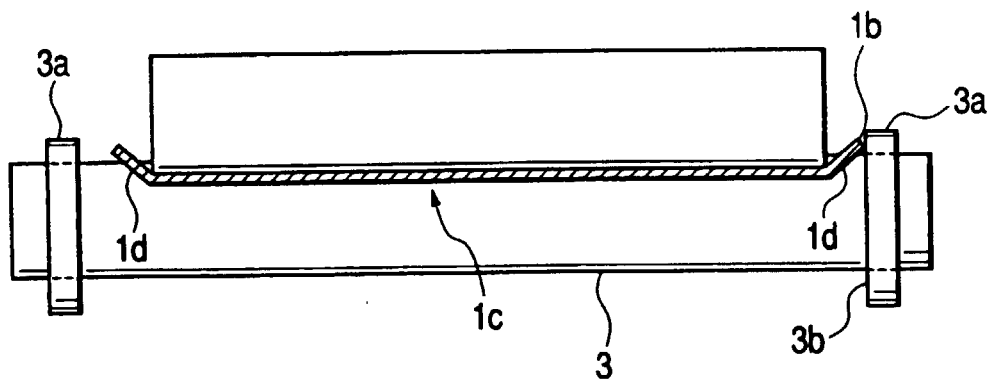
FIG. 28B
