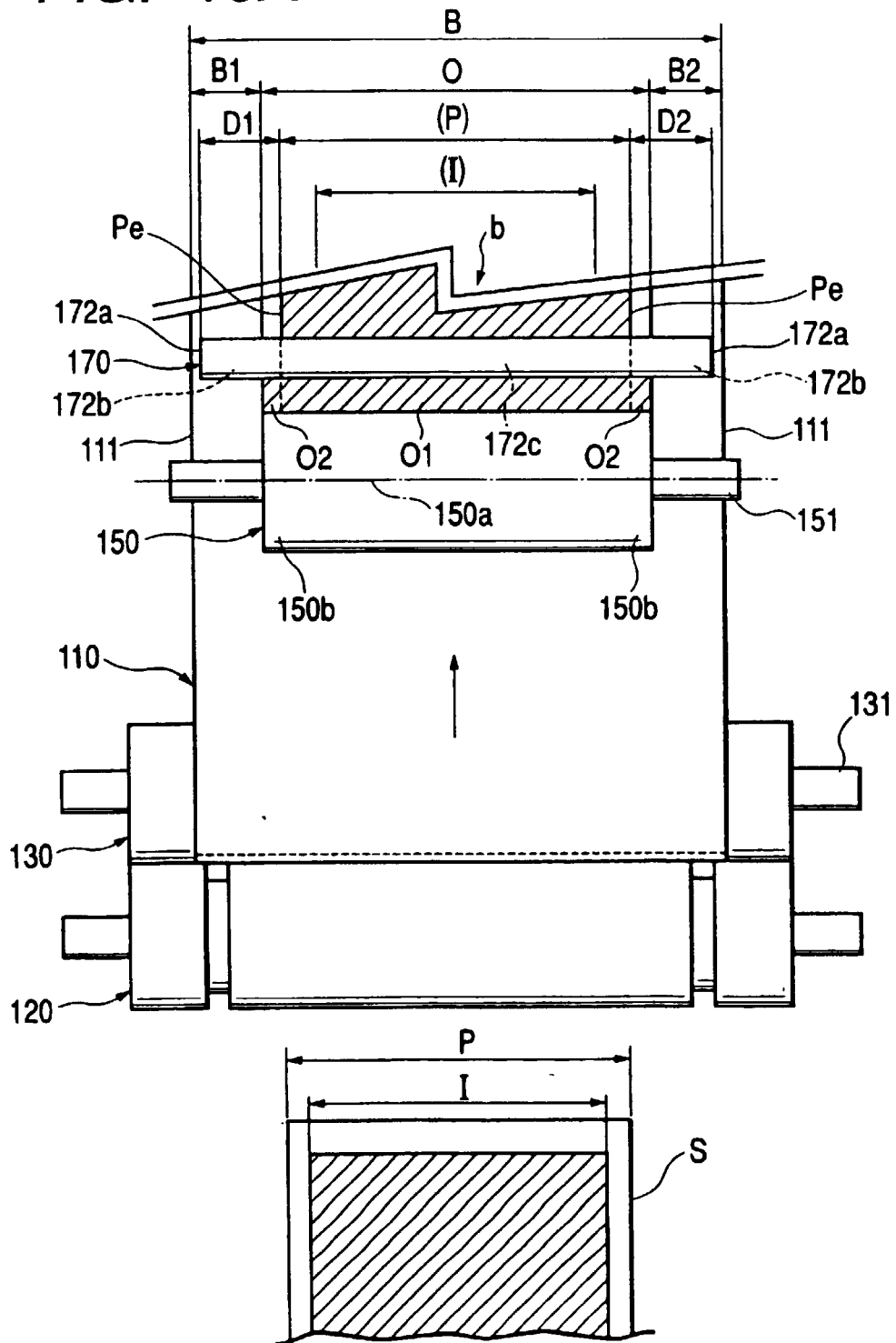
FIG. 10A
