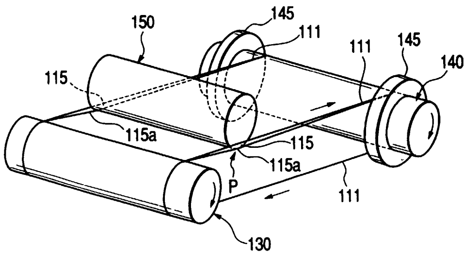
FIG. 16C
