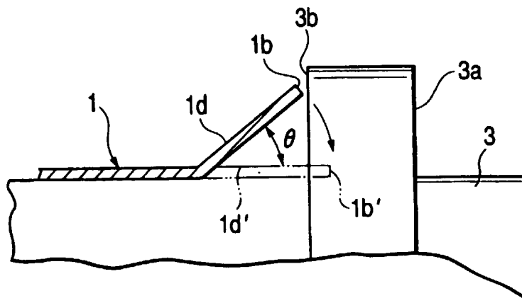
FIG. 28C
