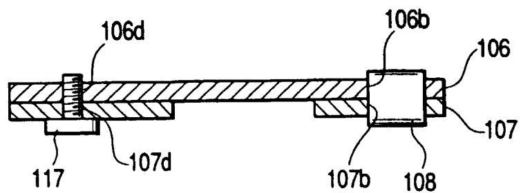
FIG. 19B
