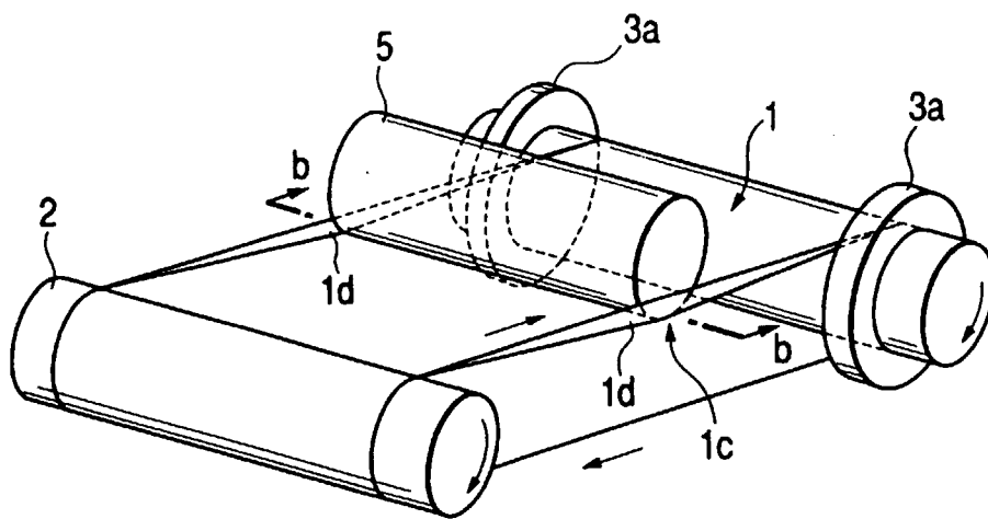
FIG. 28A
