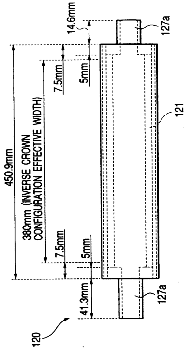
FIG. 24B
