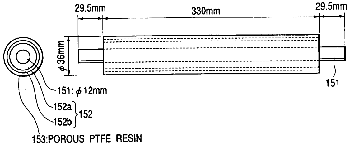
FIG. 26A
