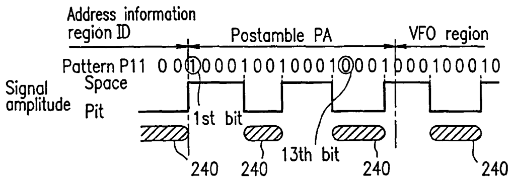
FIG. 24G Next state : 3 or 4, ID end : Mark
