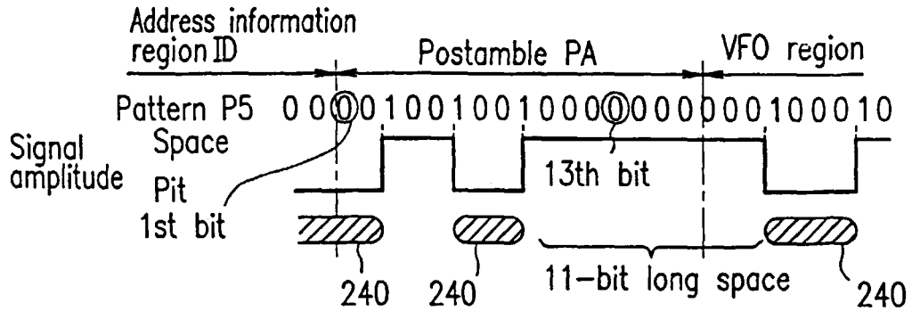
FIG. 24B Next state : 1 or 2, ID end : Space
