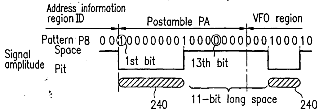
FIG. 24D Next state : 3 or 4, ID end : Space
