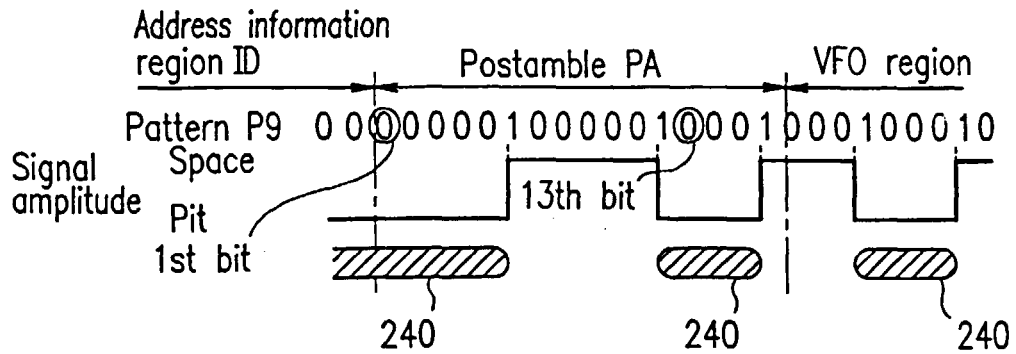
FIG. 24F Next state : 1 or 2, ID end : Space
