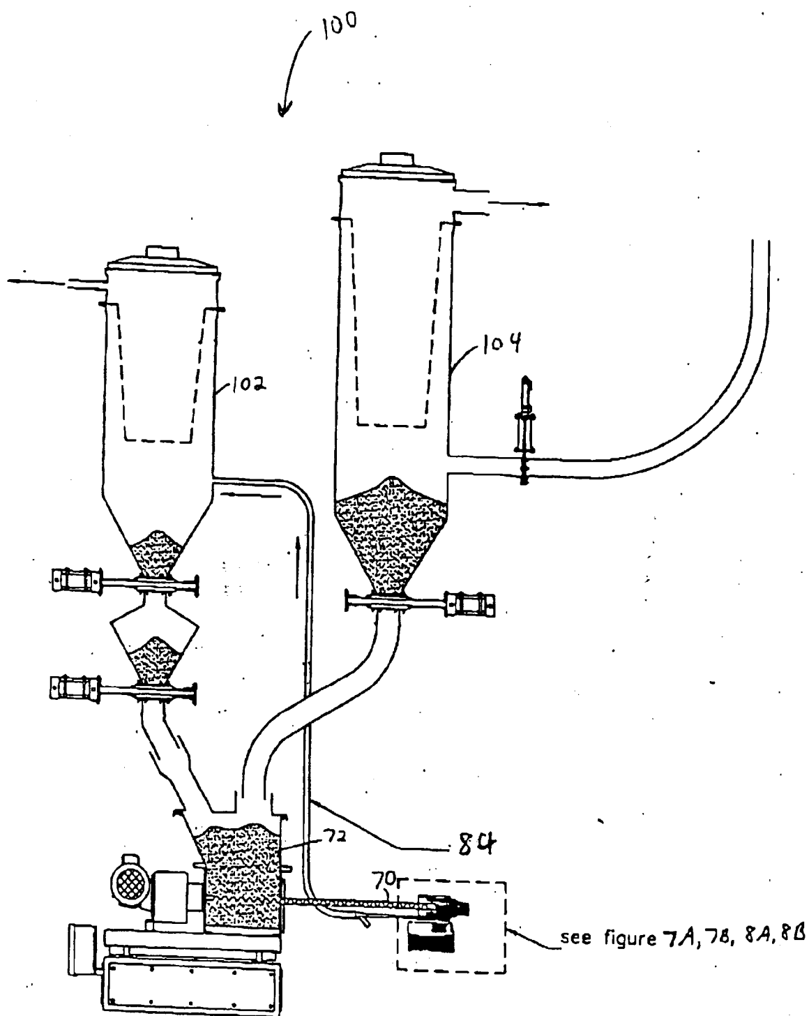
GRAVIMETRIC FEEDER
