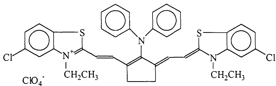
IR 140 (standard)
