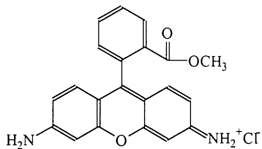
Rhodamine 123
