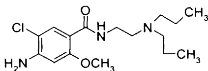
Metoclopramide
