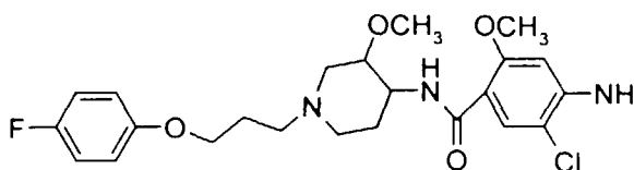
Cisapride
