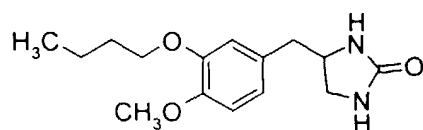
Ro 20-1724
