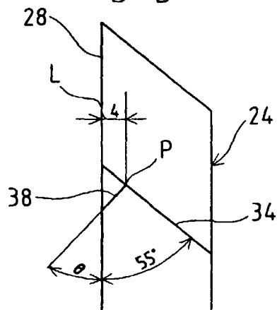
FIG. 4 (2) B - B
