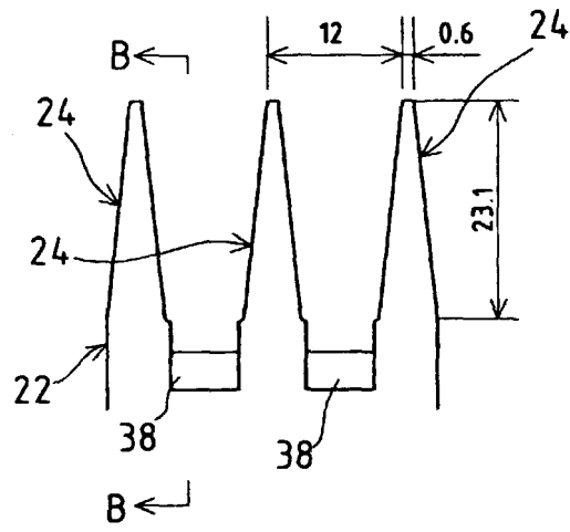
FIG. 4 (2) B - B
