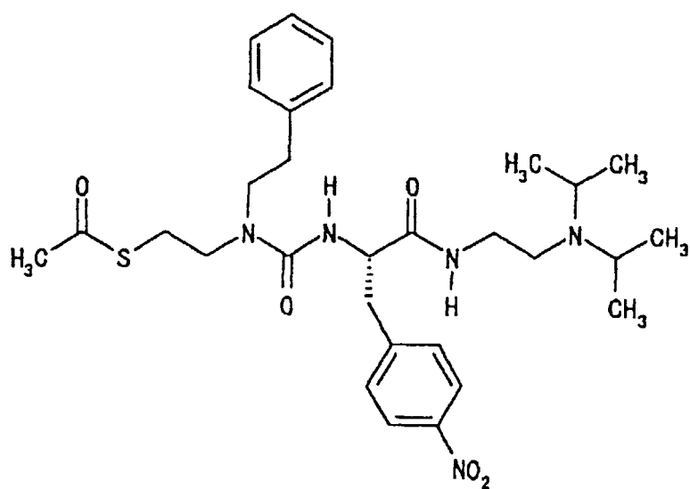
6) (2S)-2-[3-[2-(Acetylthio)ethyl]-3-phenethylureido]-N-[2-(diisopropylamino)ethyl]-3-(4-nitrophenyl)propionamide
