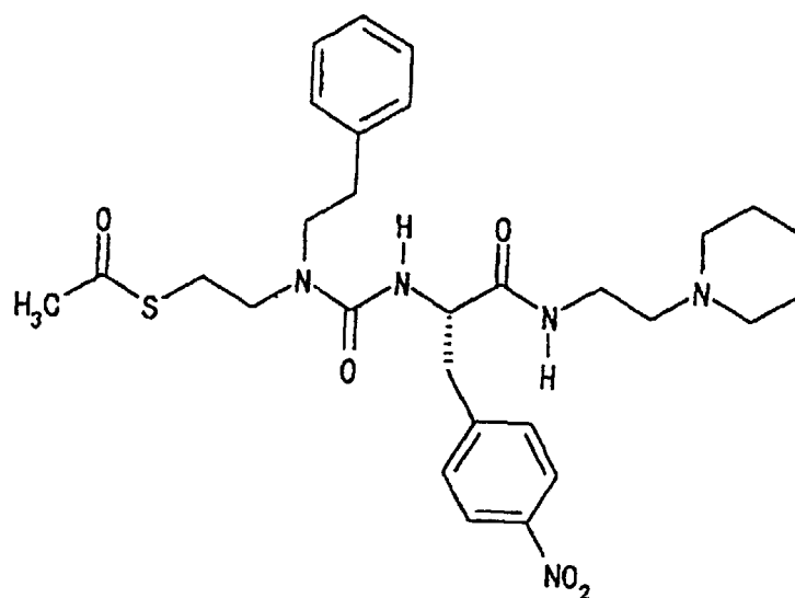
14) (2S)-2-[3-[2-(Acetylthio)ethyl]-3-phenethylureido]-3-(4-nitrophenyl)-N-[2-(piperidino)ethyl]propionamide
