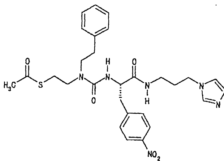
12) (2S)-2-[3-[2-(Acetylthio)ethyl]-3-phenethylureido]-N-[3-(1-imidazolyl)propyl]-3-(4-nitrophenyl)propionamide
