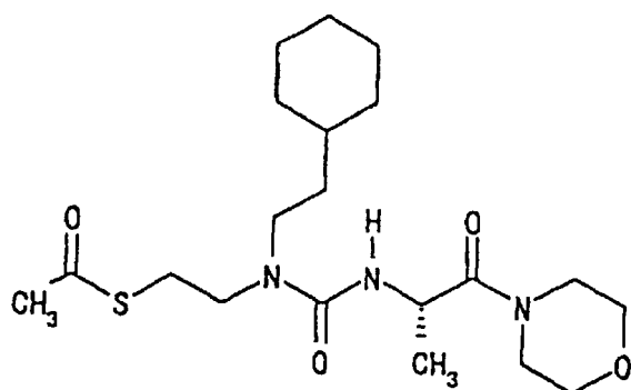
22) 4-[(2S)-2-[3-[2-(Acetylthio)ethyl]-3-henethylureido]propionyl]morpholine
