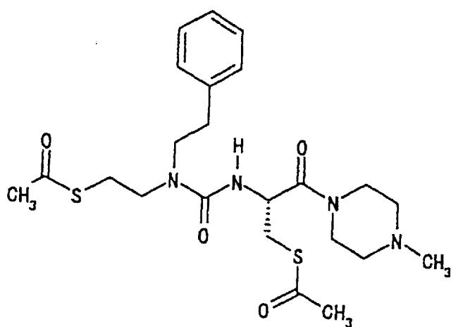
21) 1-[(2R)-3-(Acetylthio)-2-[3-[2-(acetylthio)ethyl]-3-phenethylureido]propionyl]-4-methylpiperazine
