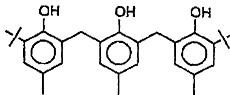
(I-32)
