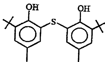
(I-28)
