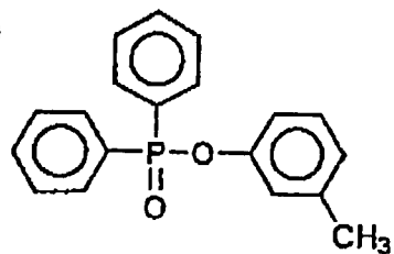
(II-22)
