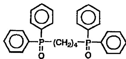
(II-13)
