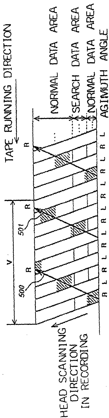
FIG. 17A
