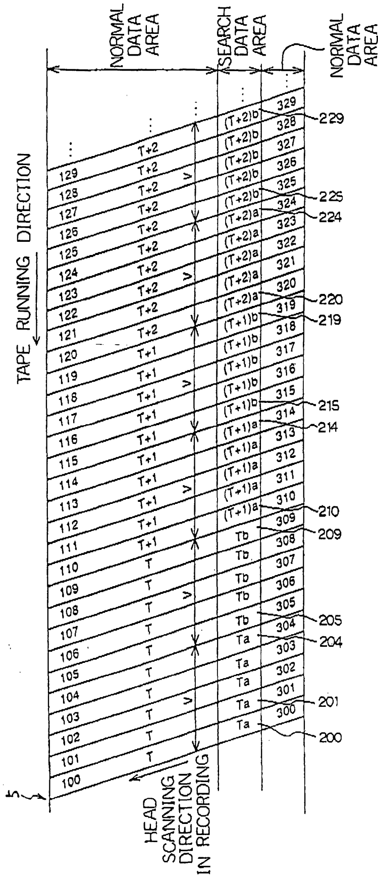
FIG. 20A
