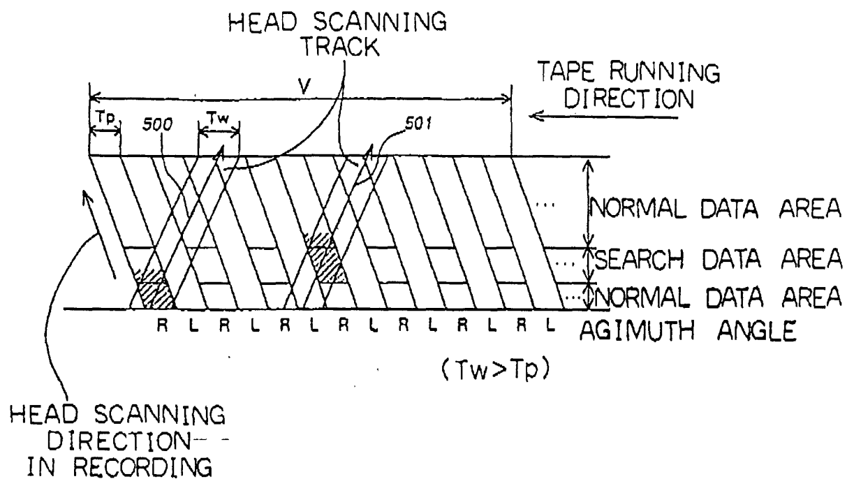
FIG. 18A
