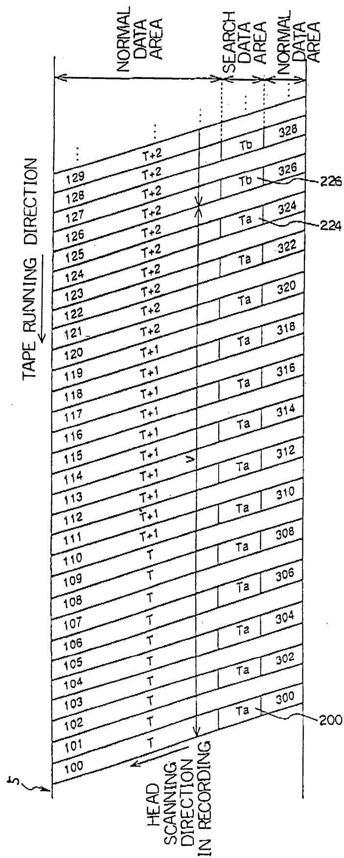
FIG. 27
