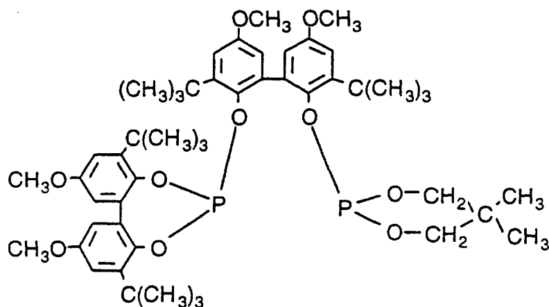
Ligand P
