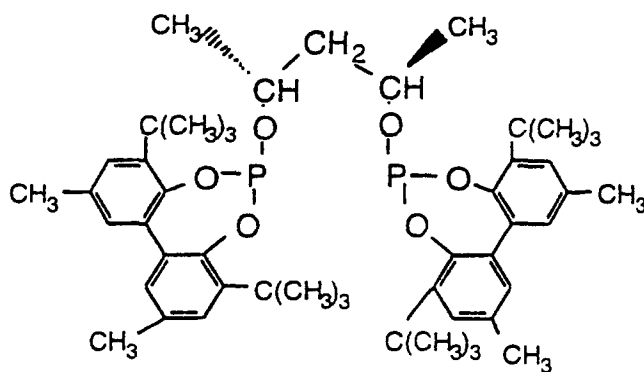
Ligand J
