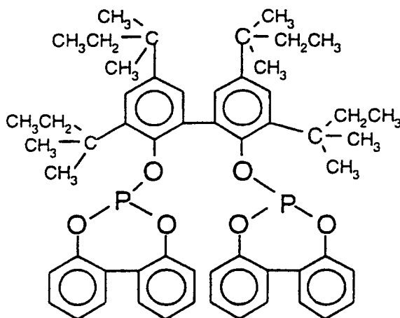
Ligand E
