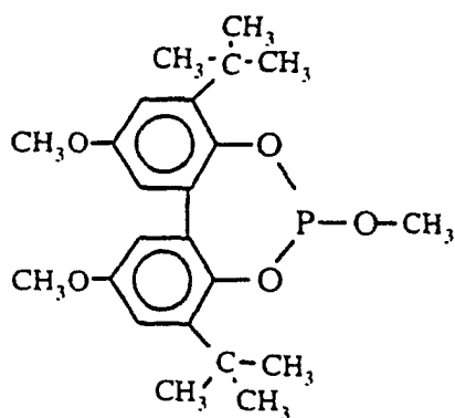
Ligand B
