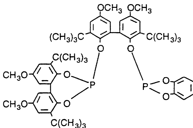
Ligand O
