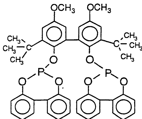
Ligand D
