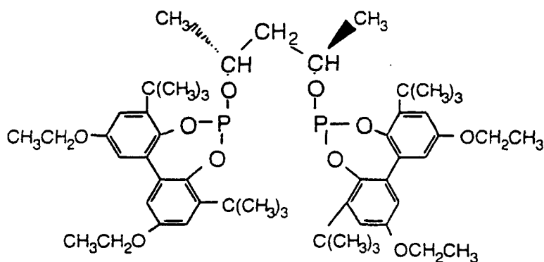
Ligand K
