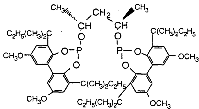
Ligand I
