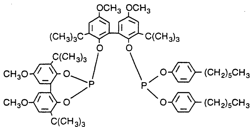
Ligand Q
