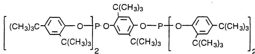
Ligand T
