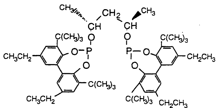
Ligand L
