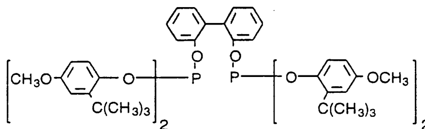
Ligand V
