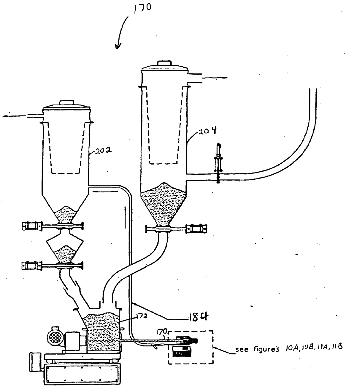
GRAVIMETRIC FEEDER
