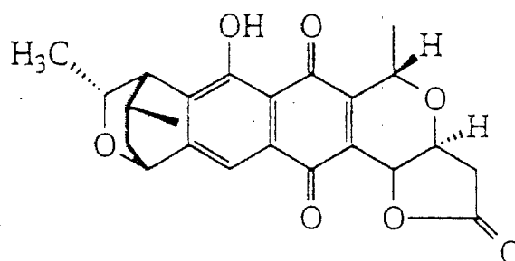
GRANATICIN (4)
