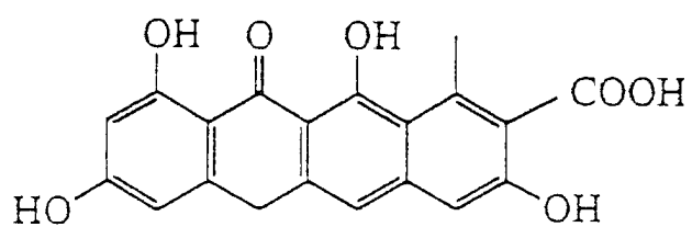
TETRACENOMYACIN F1 (5)
