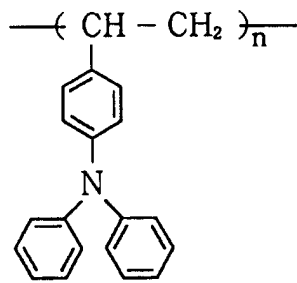
DPA - PS
