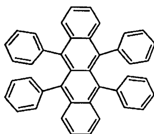
Rubrene
