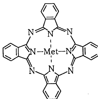
Met - Pc
