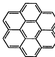
Coronene
