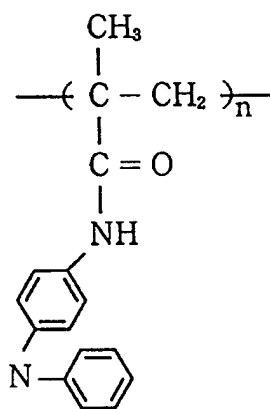
TPD - PMAA
