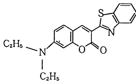
Coumarin 6
