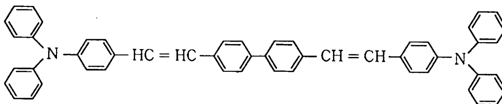
DTPABVi
