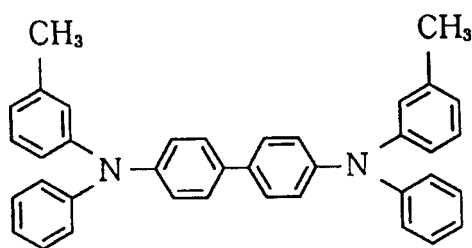
TPD
