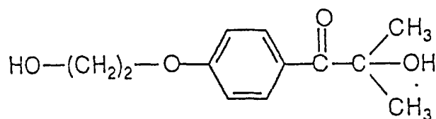
Unmodified DARCUR 2959 ®
