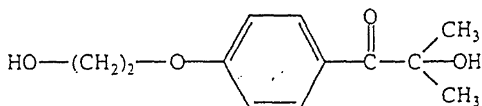
2959
