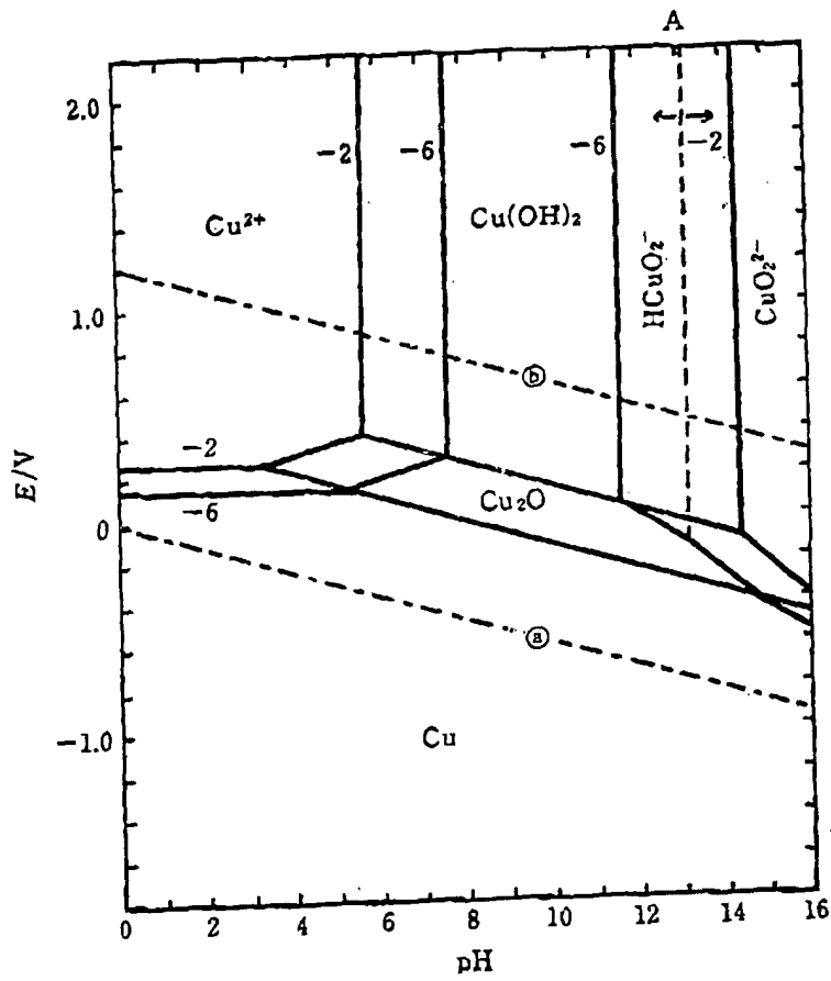
Pourbaix Diagram: Cu-H 2 O system (25°C)
